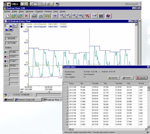
Curva de consumo de una población. Funciones máximo, medio y mínimo diarios
